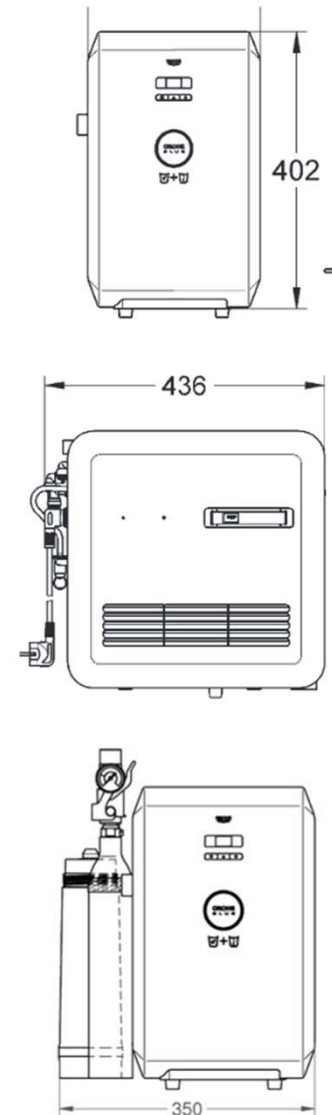
Größen des Kühlers/Karbonisators
